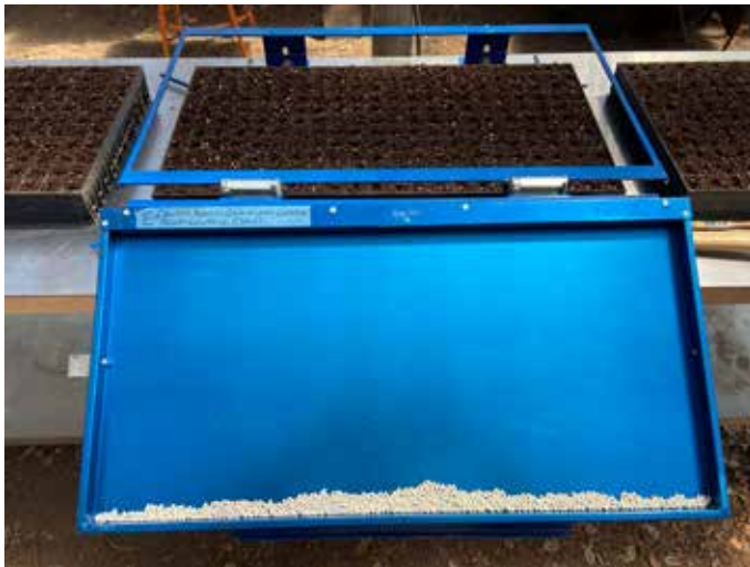
FIGURA 15. Plato de la sembradora de vacío con semillas recubiertas de lechuga, sueltas antes de su distribución a cada hoyo.
